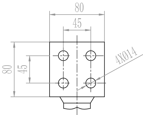
低压接线端子
