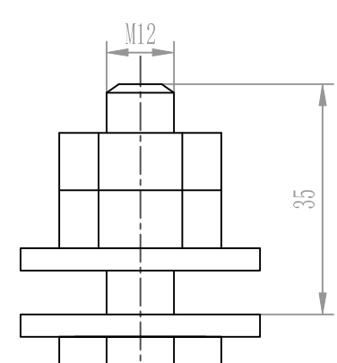
低压零相接线端
